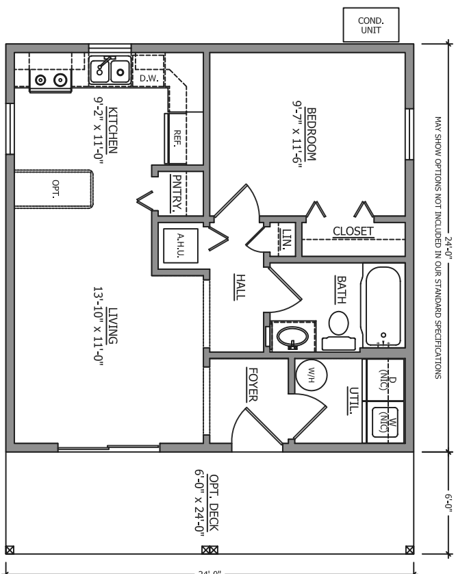
FLOOR PLAN N.T.S.
